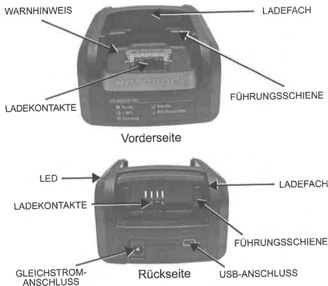
Abb.1 Akkuladegerät
